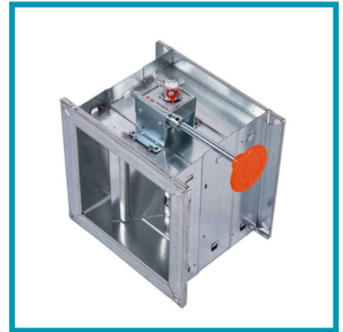
VAN TAY VẶN | VOLUME CONTROL DAMPER (GEAR BOX)
